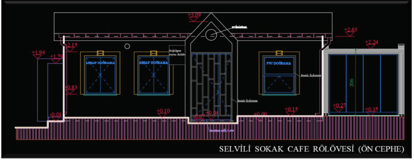
Selvili Sokak kafe rölövesi – ön cephe
